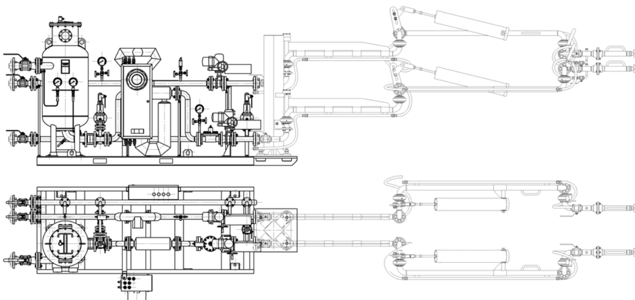
Рисунок 1 – Установка УИЖГЭ в составе с комплексом СГСН – 50/50.
