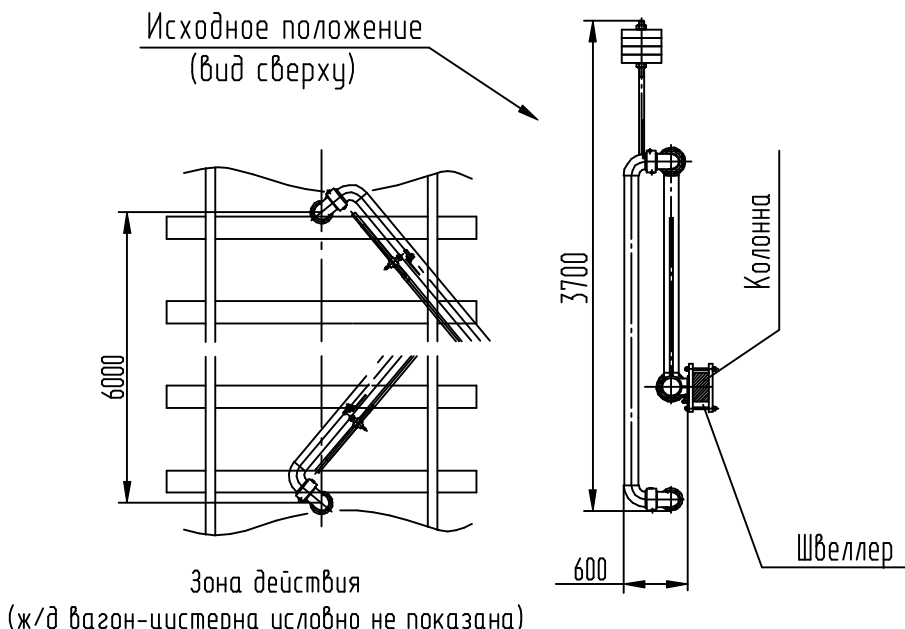
Монтажная схема
