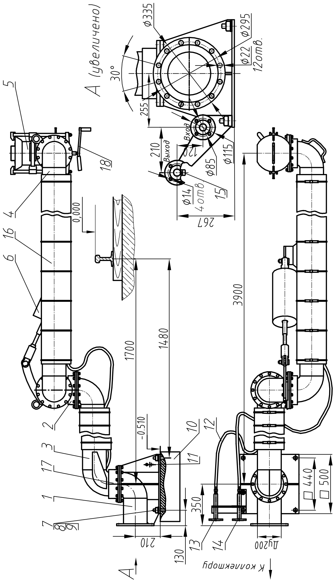
Устройство УСН-200П-06 с зоной действия 6м.
