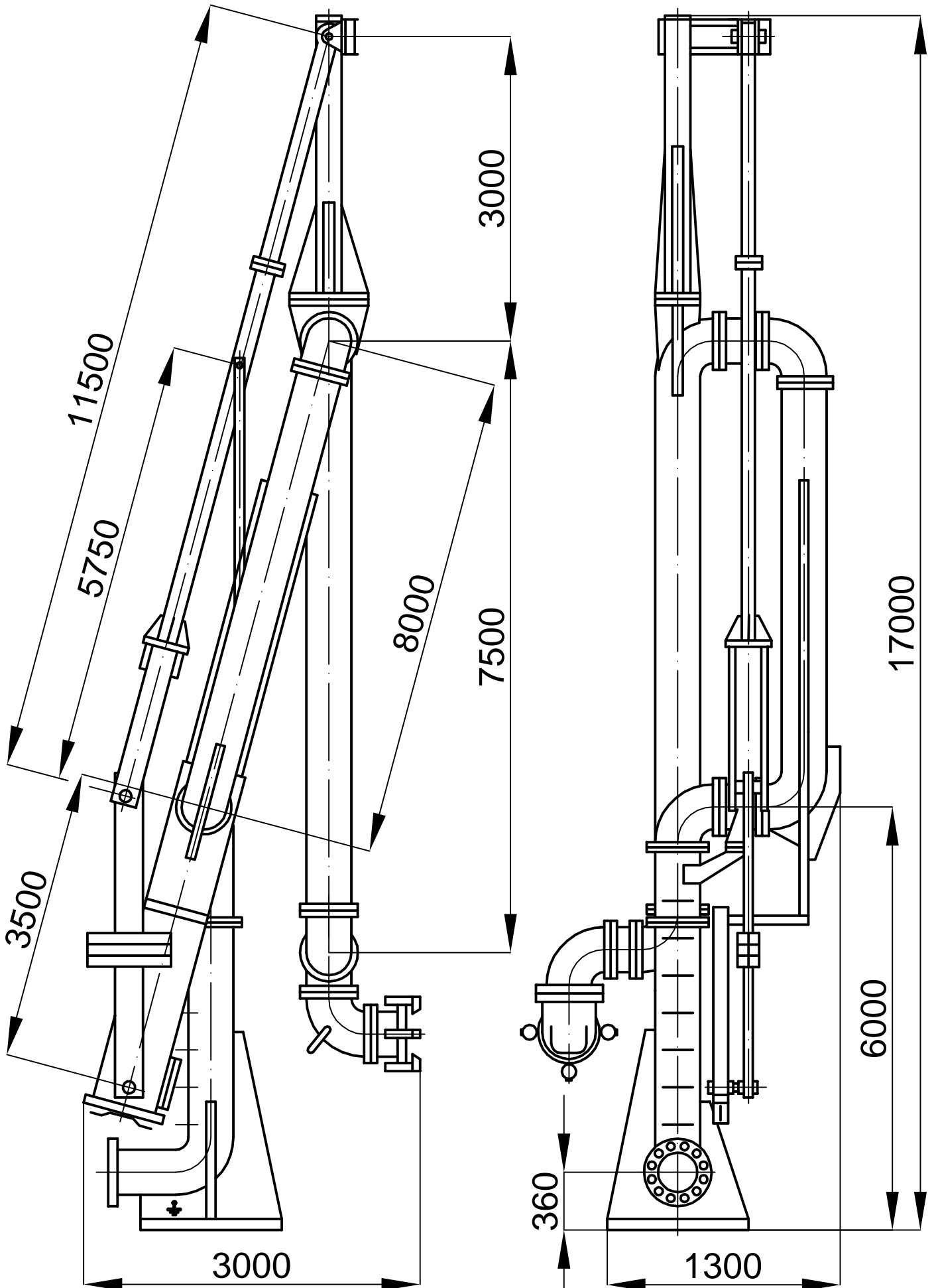
Рисунок 3- Стендер СР-250-03
