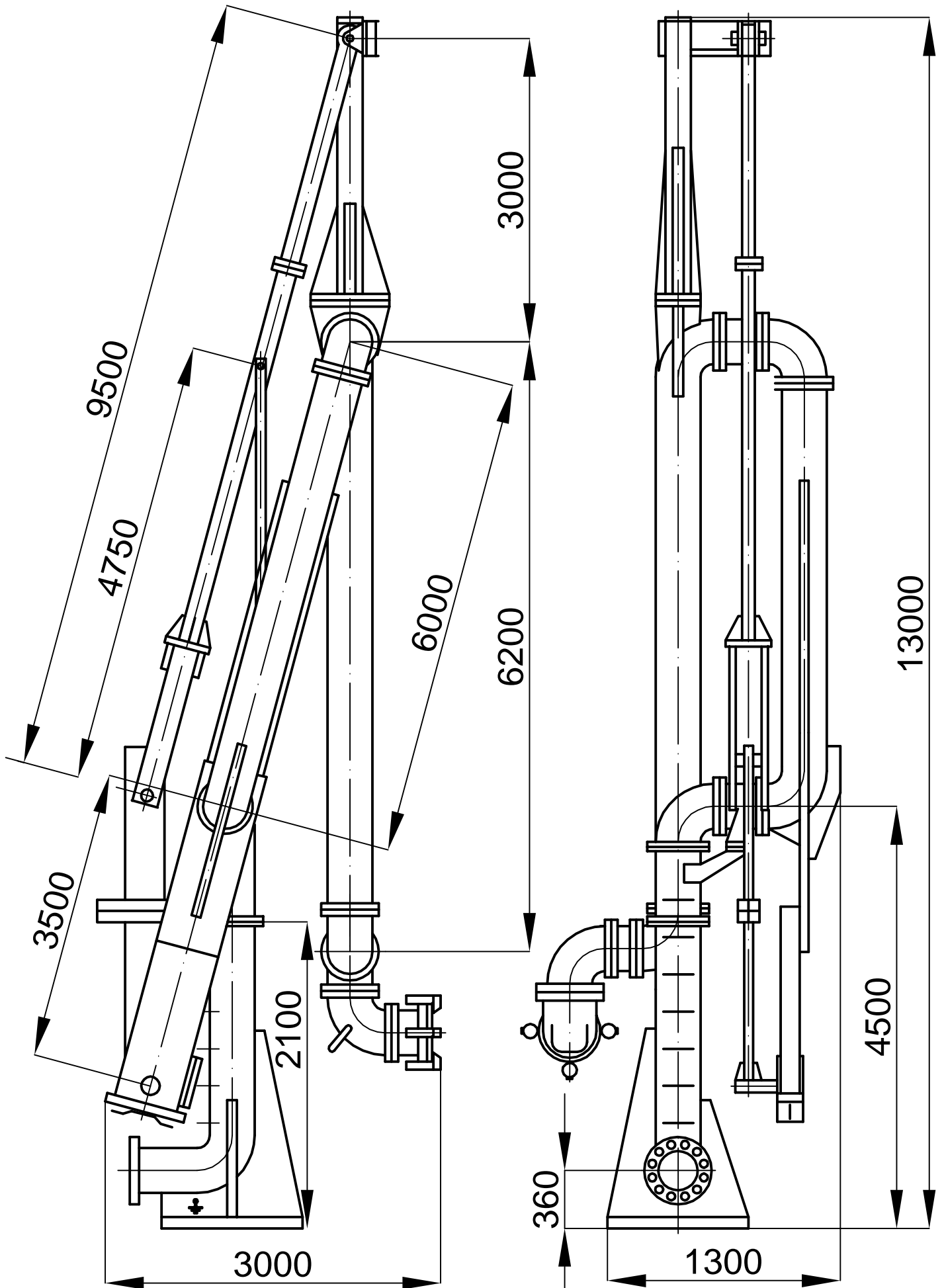
Рисунок 2- Стендер СР-250-02
