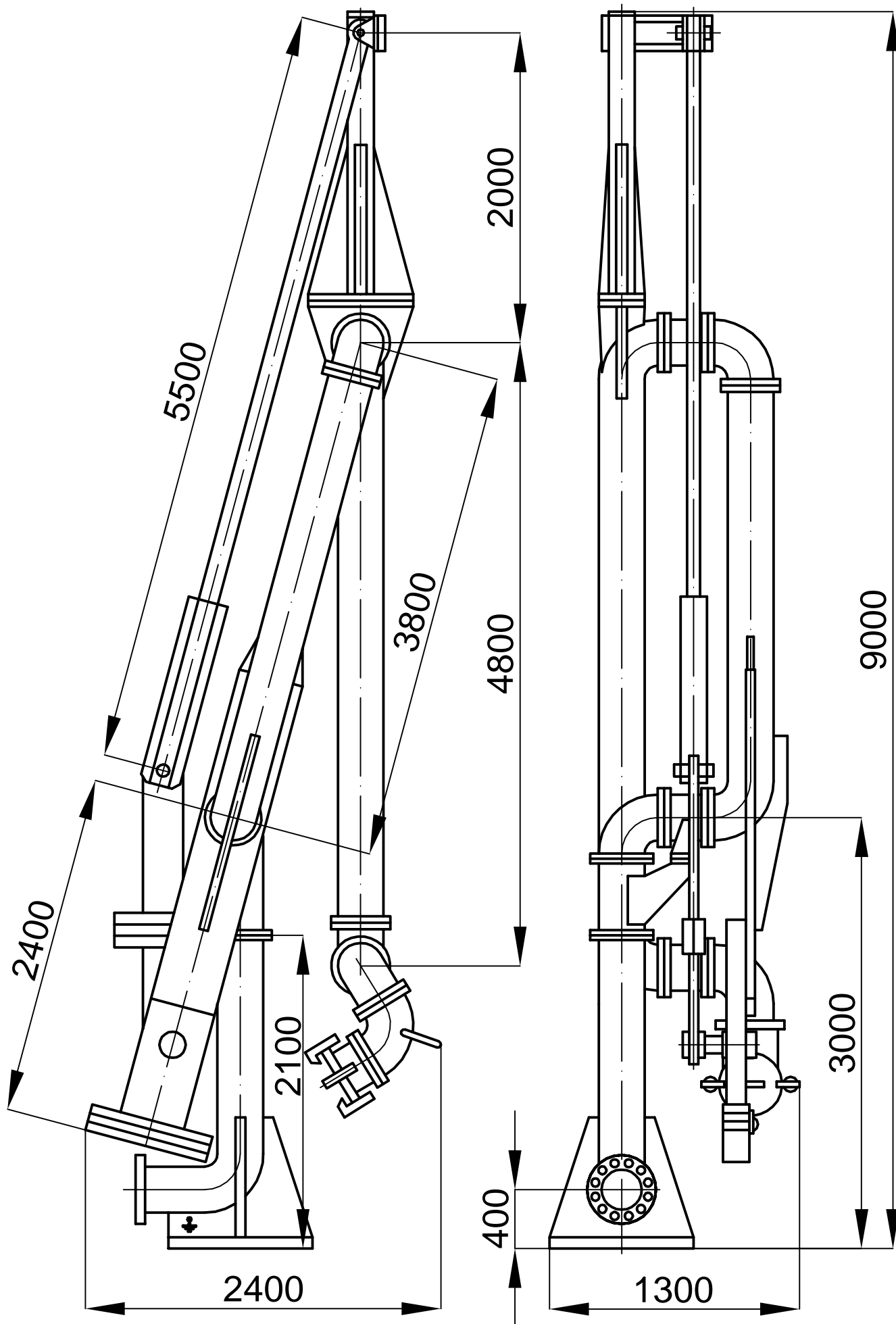
Рисунок 1- Стендер СР-250-01
